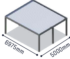
3 raylı 1 sistem maksimum ölçüler
